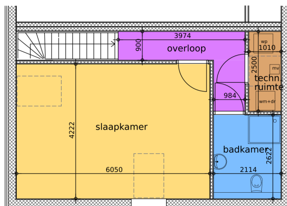
Appartement 24 G.O.=43,4 m2 eerste verdieping
