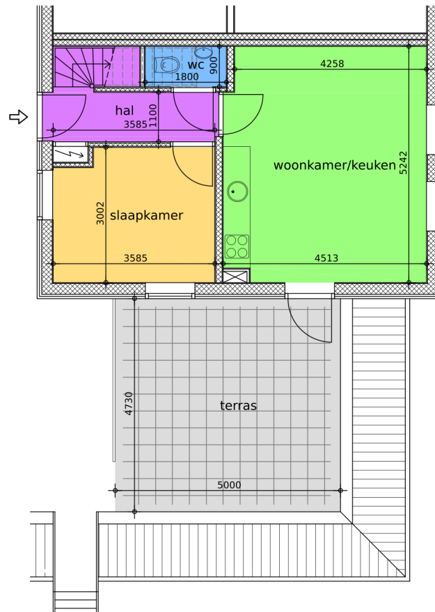
Appartement 24 G.O.=43,4 m2 eerste verdieping
