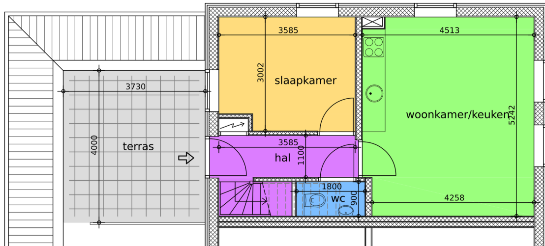
Appartement 23 G.O.=43,4 m 2 eerste verdieping
