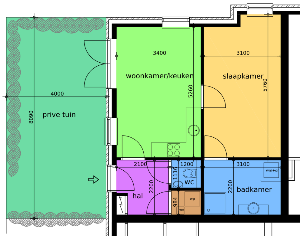
Appartement 19 G.O. = 50,7 m 2
